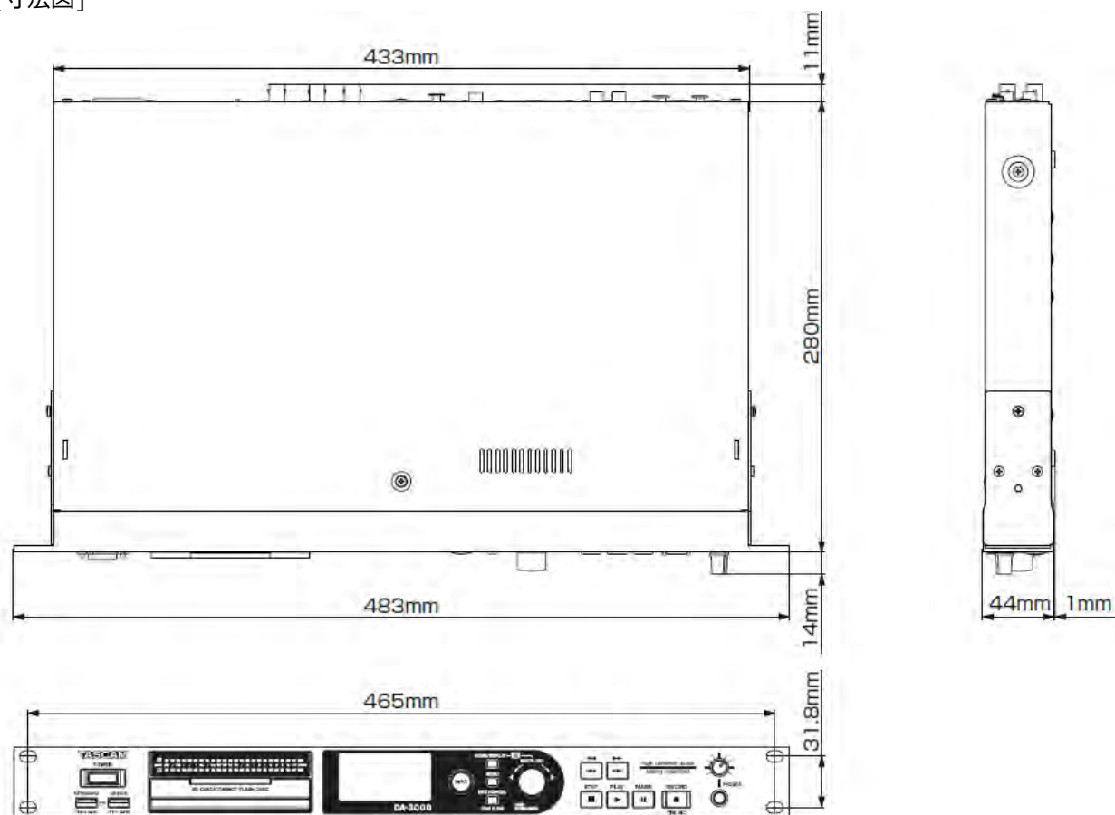
[寸法図]
